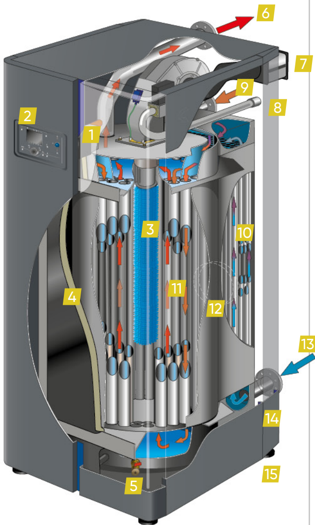
PRZEKRÓJ KOTŁA
