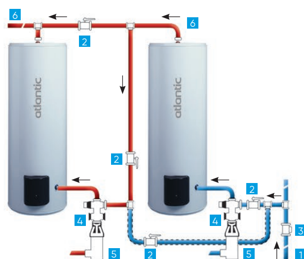
schemat uniwersalnego podłączenia hydraulicznego ogrzewacza dużej pojemności o konstrukcji stojącej, umożliwiający zasilanie jednego lub obu urządzeń (szeregowo lub równolegle)
