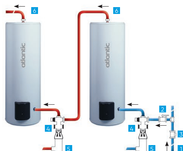
schemat szeregowego podłączenia hydraulicznego ogrzewacza dużej pojemności o konstrukcji stojącej
