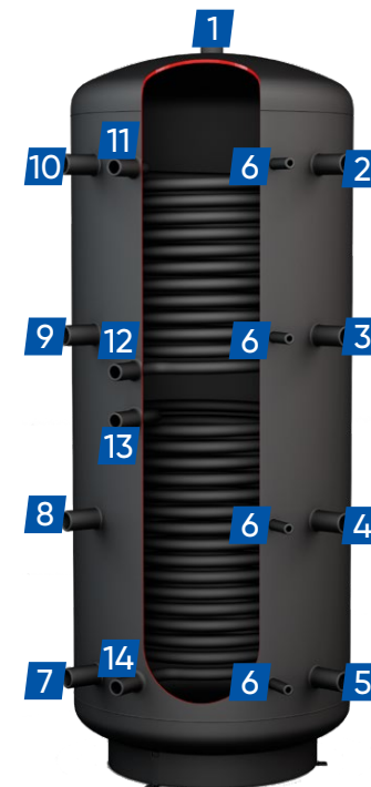
PRZEKRÓJ BUFORA
